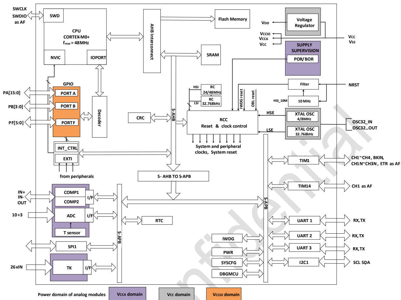
图 1-1 功能模块
