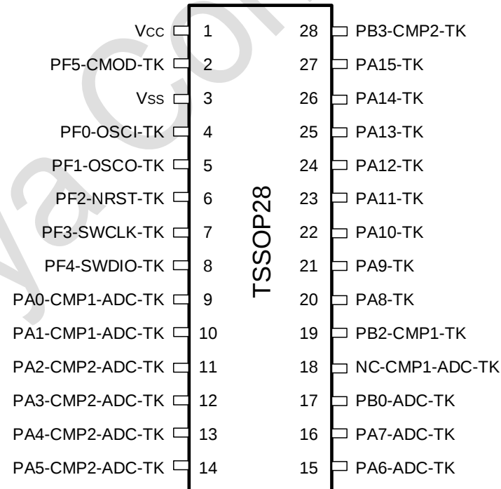
图 3-2 TSSOP28 Pinout4 PY32T020G4xP7-B (Top view)
