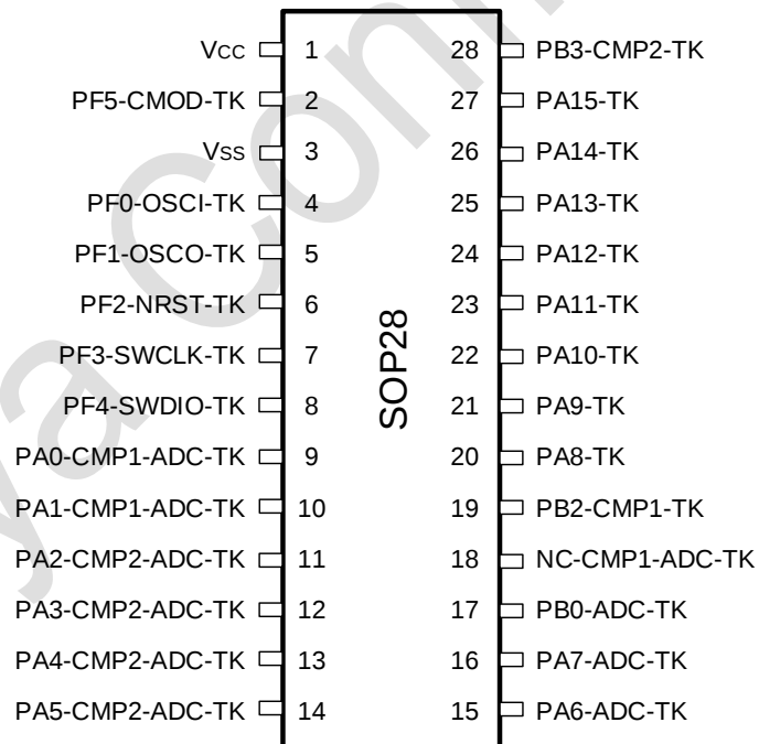
图 3-6 SOP28 Pinout4 PY32T020G4xS7-B (Top view)
