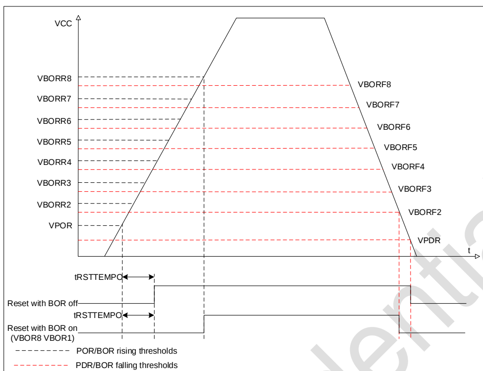
图 2-3 POR/PDR/BOR 阈值
