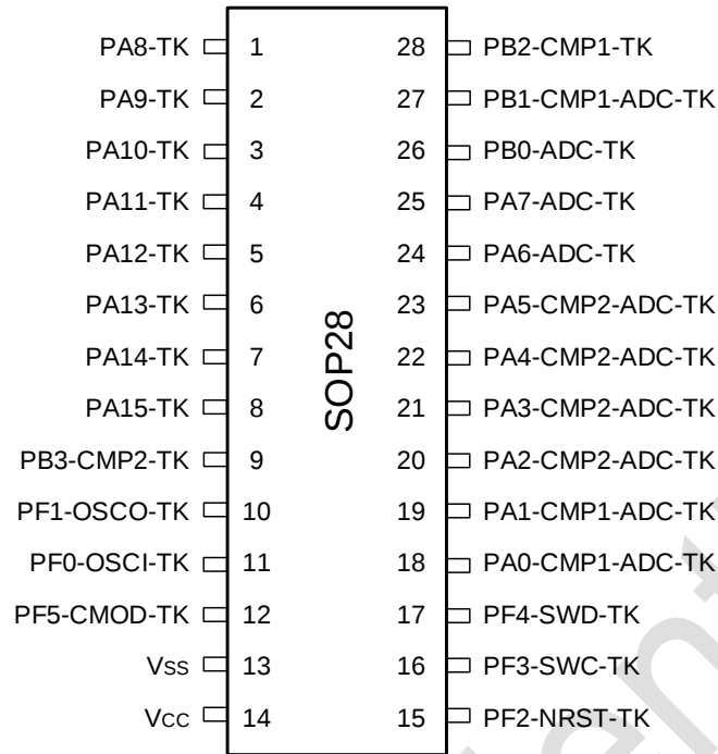
图 3-5 SOP28 Pinout3 PY32T020G3xS7-B (Top view)
