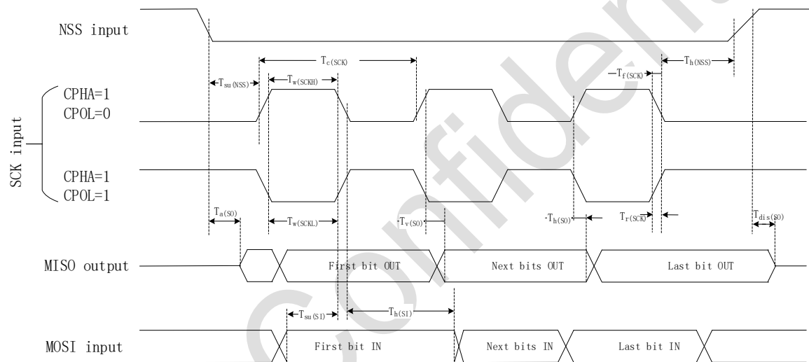
图 5-5 SPI 时序图-从机模式和 CPHA=1
