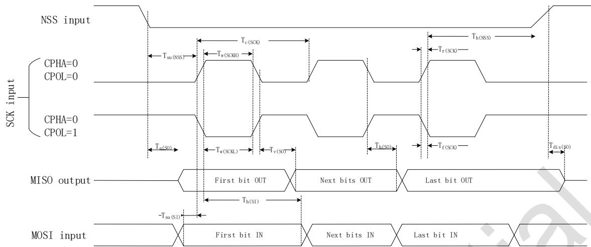
图 5-4 SPI 时序图-从机模式和 CPHA=0
