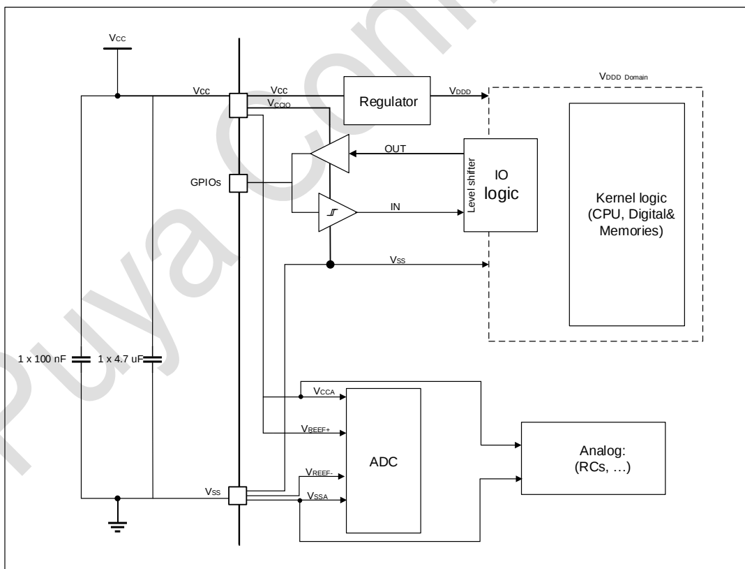
图 5-1 供电方案图
