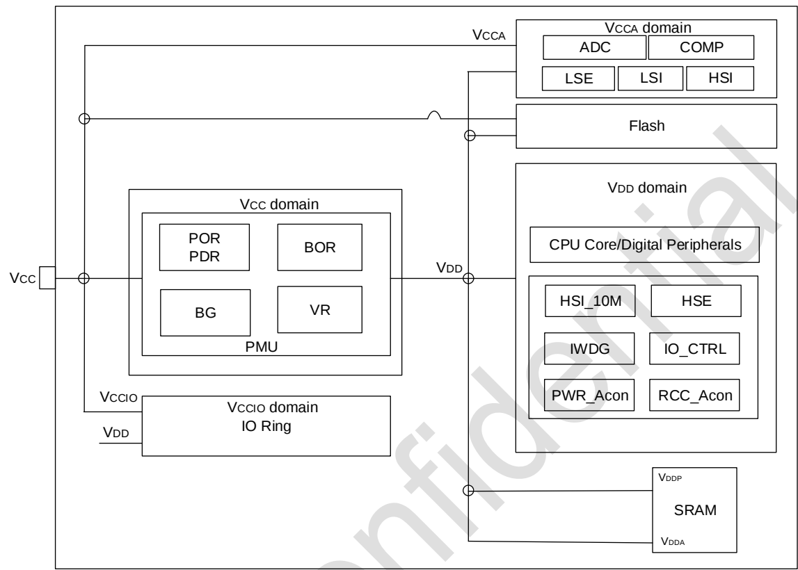
图 2-2 电源框图
