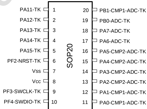
图 3-9 SOP20 Pinout2 PY32T020F2xS7-B (Top view)
