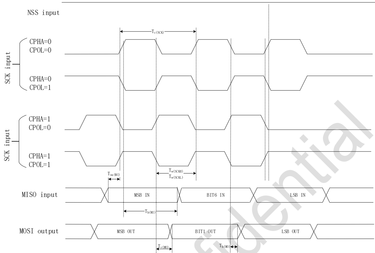
图 5-6 SPI 时序图-主机模式
